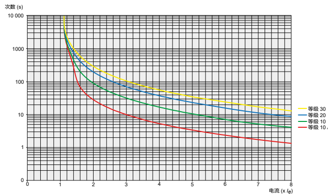
集成电子过载保护的脱扣曲线
